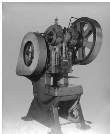
镇海锻压机床厂制造的 60T 压力机
